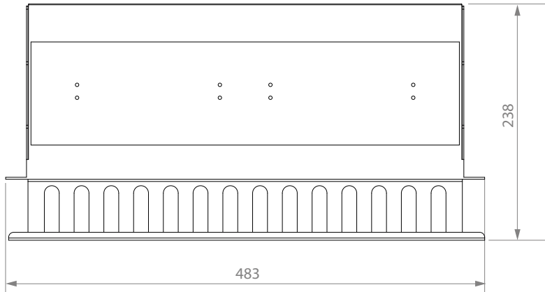
REF. 9D.FO159-12SC MOD SMT 3U 7TE 12SC/E2000 + ADAPT+PIGT+NUMER
