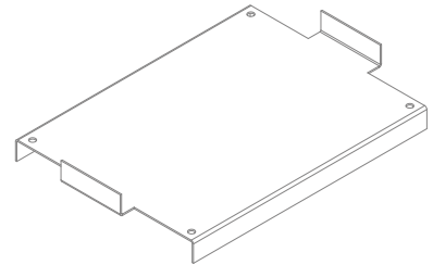
REF. 9D.FOCasM-02 Cassette INTERMEDIA Emp. mod. metálico
