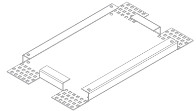
REF. 9D.FOCasM-01 Cassette BASE Emp. mod. metálico 250x138x15mm
