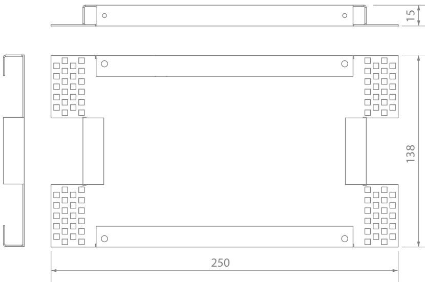
REF. 9D.FOCasM-01 Cassette BASE Emp. mod. metálico 250x138x15mm
